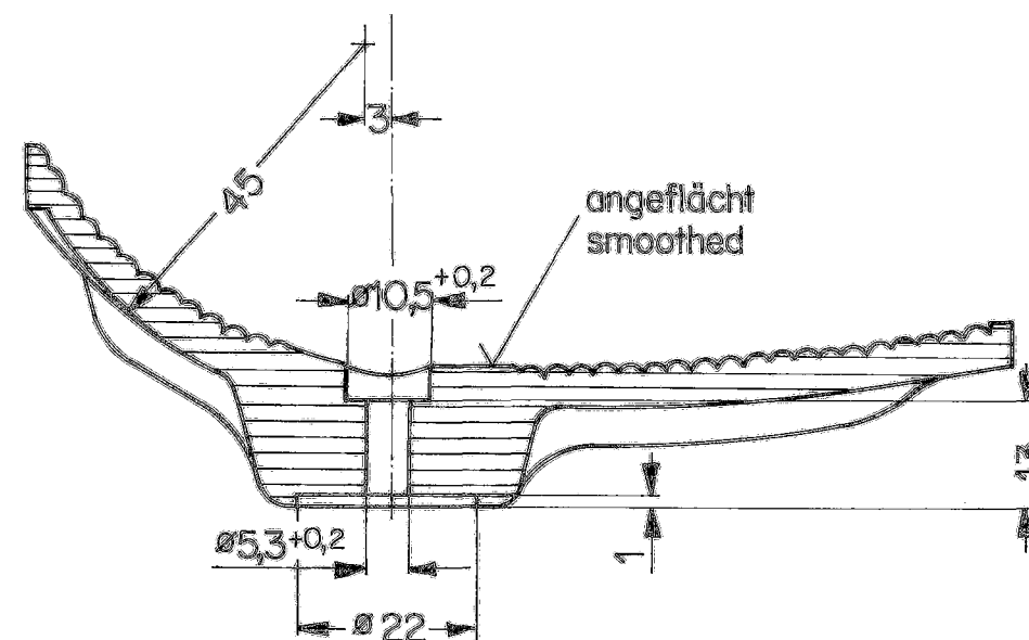
Schnitt Section A-B
