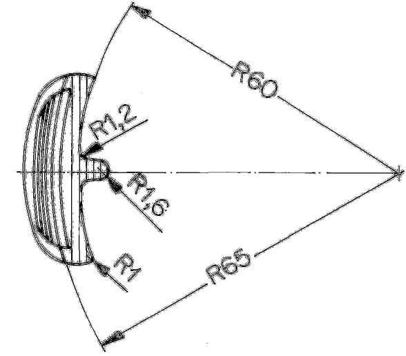
Schnitt Section I-K
