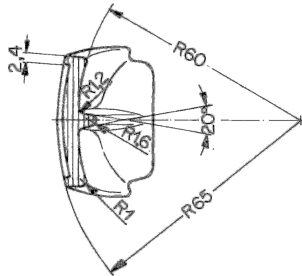
Schnitt Section E-F
